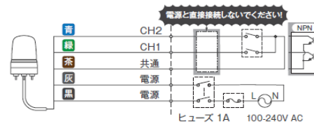
M2KT (AC100-240V / 2点穴式取付・プッシュイン端子台)
