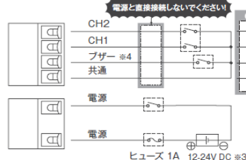
M1KT (DC12-24V / 2点穴式取付・プッシュイン端子台)
