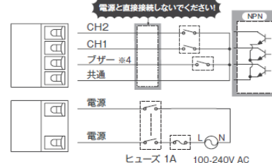
M2KT (AC100-240V / 2点穴式取付・プッシュイン端子台)
